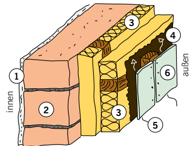
Einschaliges Mauerwerk mit hinterlüfteter Fassade
