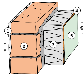
Einschaliges Mauerwerk mit Wärmedämmverbundsystem
