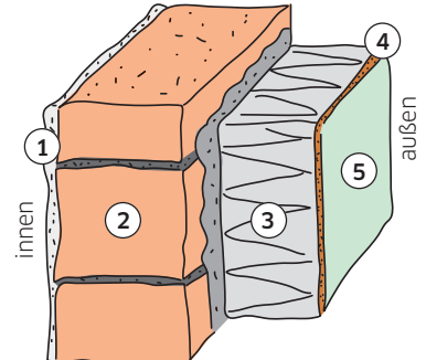
Einschaliges Mauerwerk mit Wärmedämmverbundsystem
