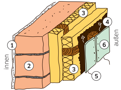
Einschaliges Mauerwerk mit hinterlüfteter Fassade
